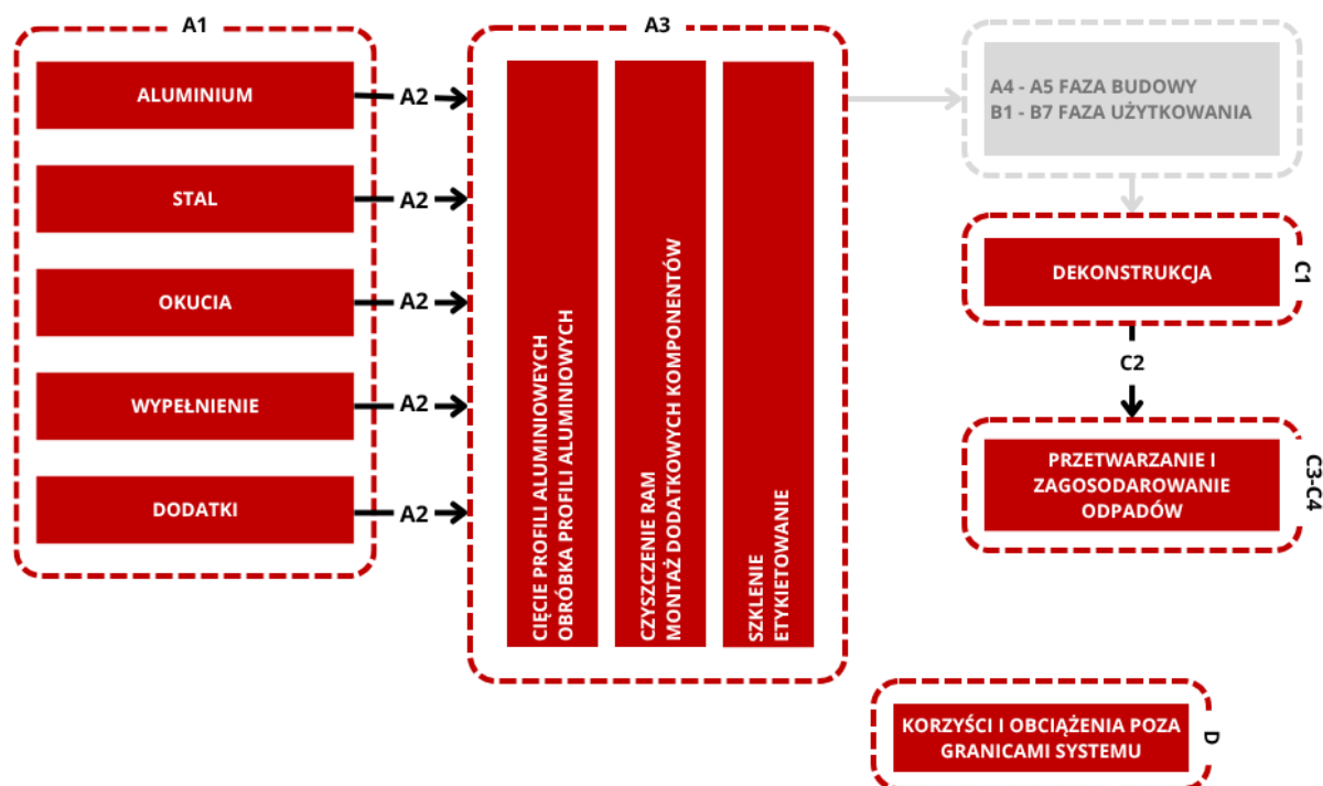
Rysunek 5.1: Granice systemu dla charakterystyki środowiskowej drzwi aluminiowych
